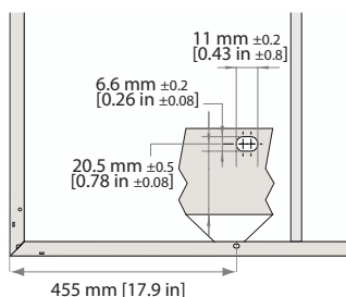
Fig. 3 Orificios de montaje: Paneles REC Alpha
