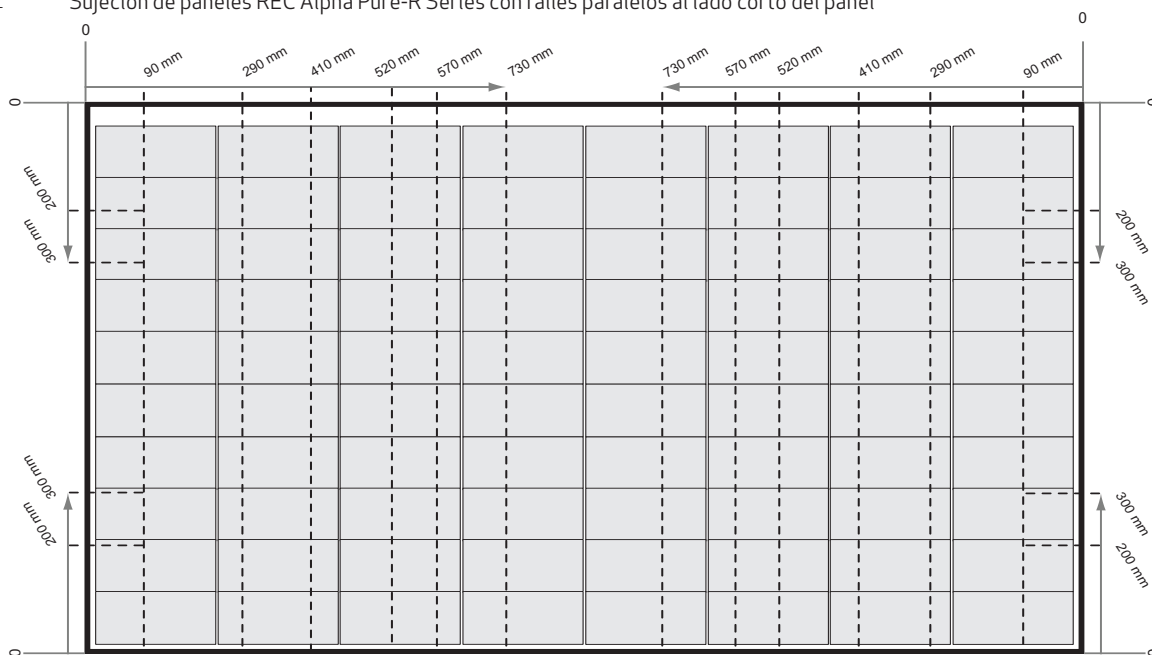
Fig. 4-1 Sujeción de paneles REC Alpha Pure-R Series con raíles paralelos al lado corto del panel
