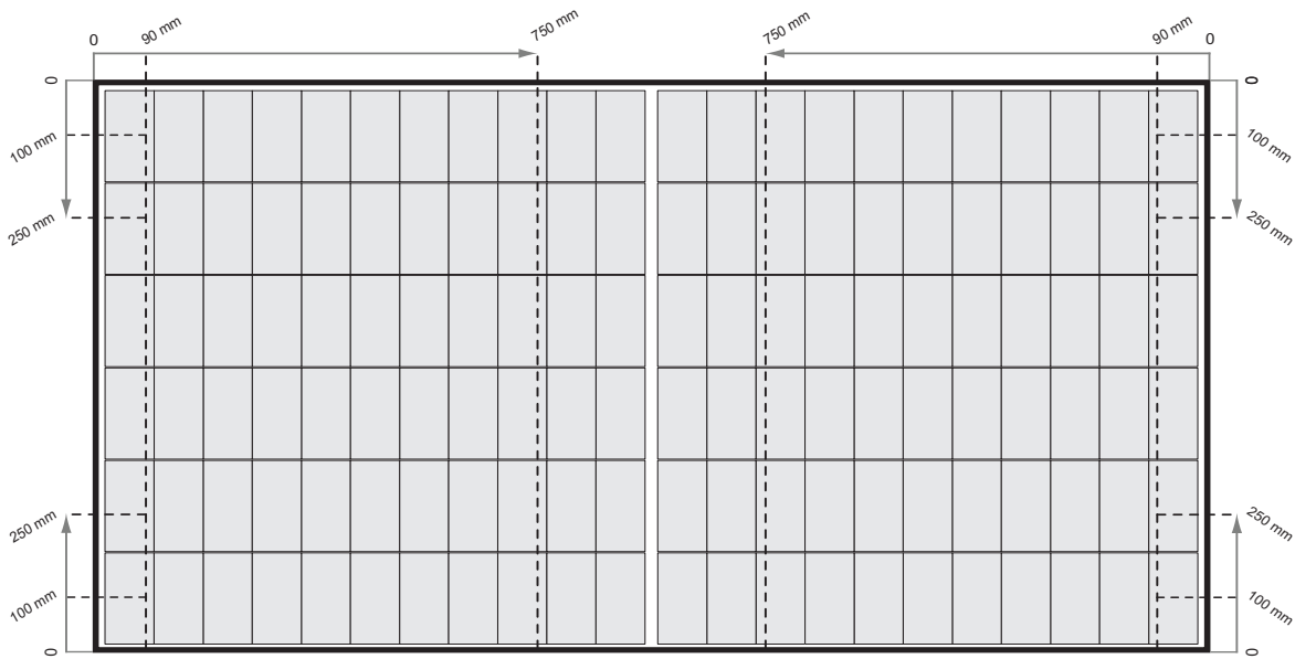
Fig. 3-2 Sujeción de paneles REC Alpha Pure 2 Series con railes paralelos al lado largo del panel
