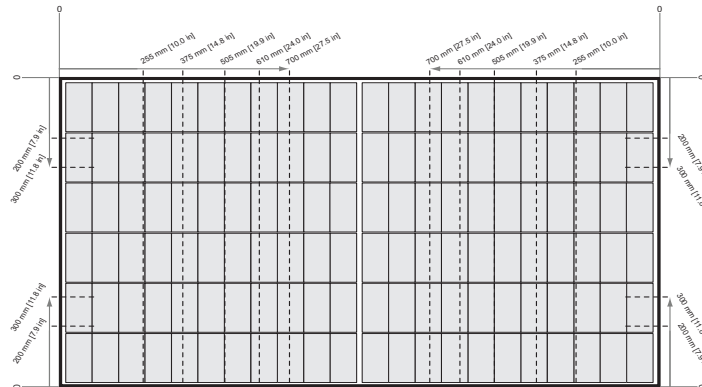
Fig. 2-3 Sujeción de los paneles REC Alpha Pure Series mediante raíles cortos
