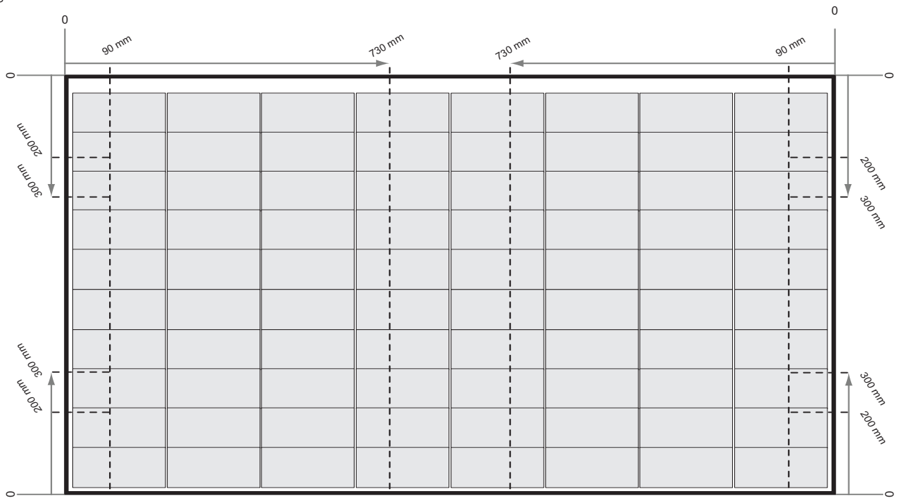
Fig. 4-2 Sujeción de los paneles REC Alpha Pure-R Series con raíles paralelos al lado largo del panel
