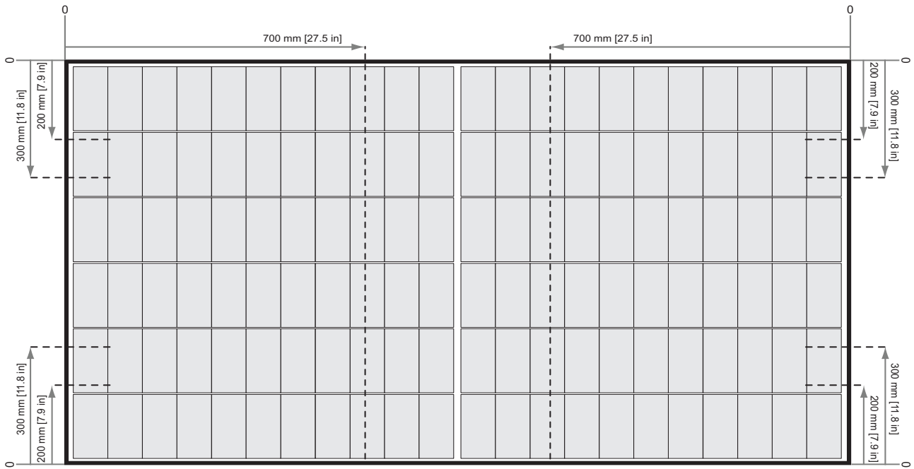
Fig. 2-2 Sujeción de paneles REC Alpha Pure Series con raíles paralelos al lado largo del panel
