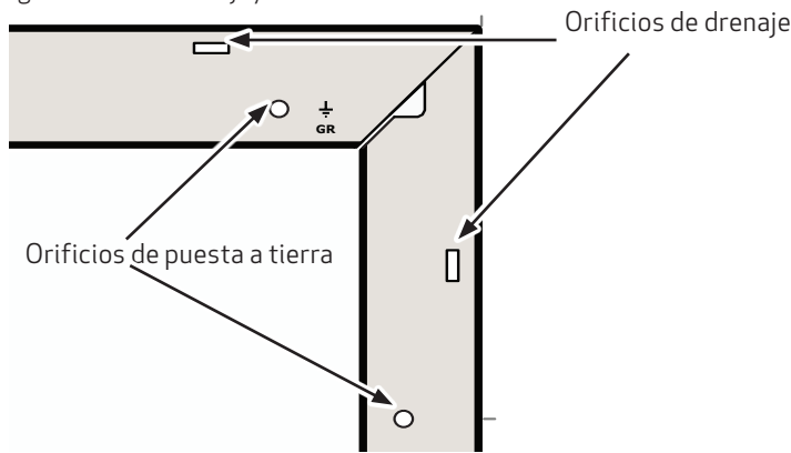
Fig. 5 Orificios de drenaje y conexión a tierra
