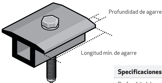
Fig. 1 Especificaciones de la abrazadera
