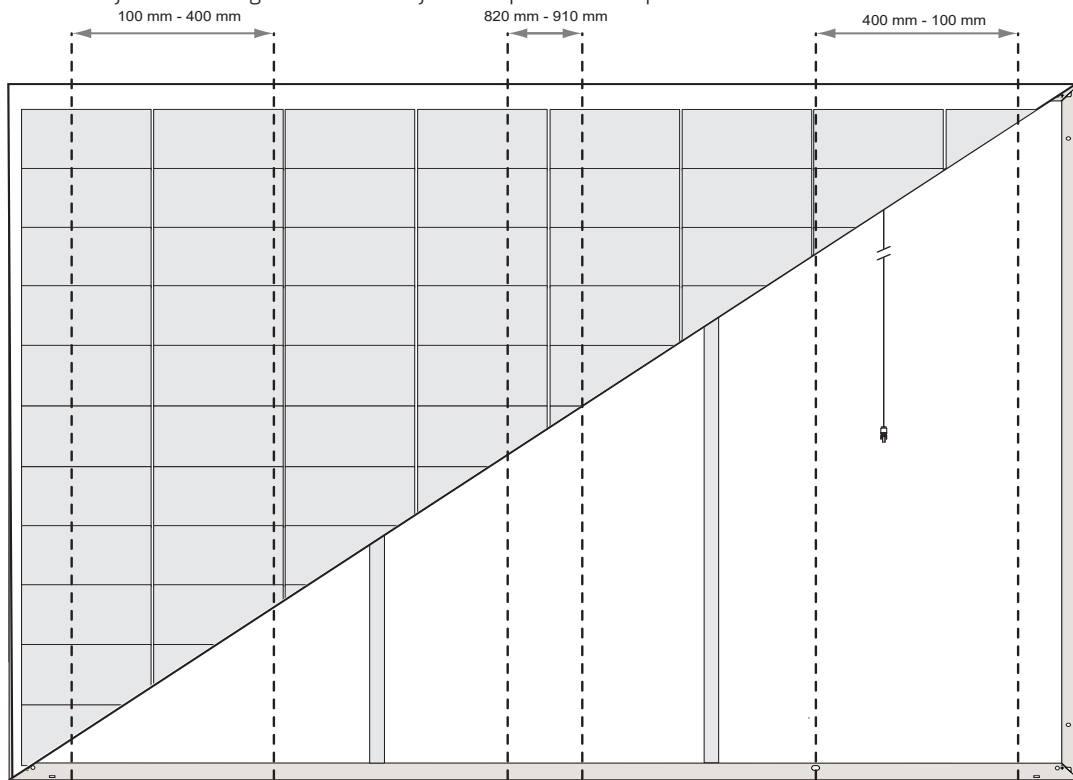
Fig. 5-4 Zonas de sujeción de configuración de montaje de seis puntos: REC Alpha Pure-RX Series
