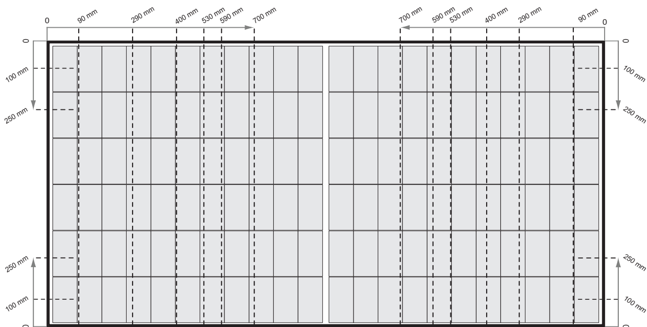
Fig. 3-1 Sujeción de paneles REC Alpha Pure 2 Series con ralles paralelos al lado corto del panel
