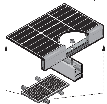
Fig. 4 Ejemplo de instalación de orificios de montaje
