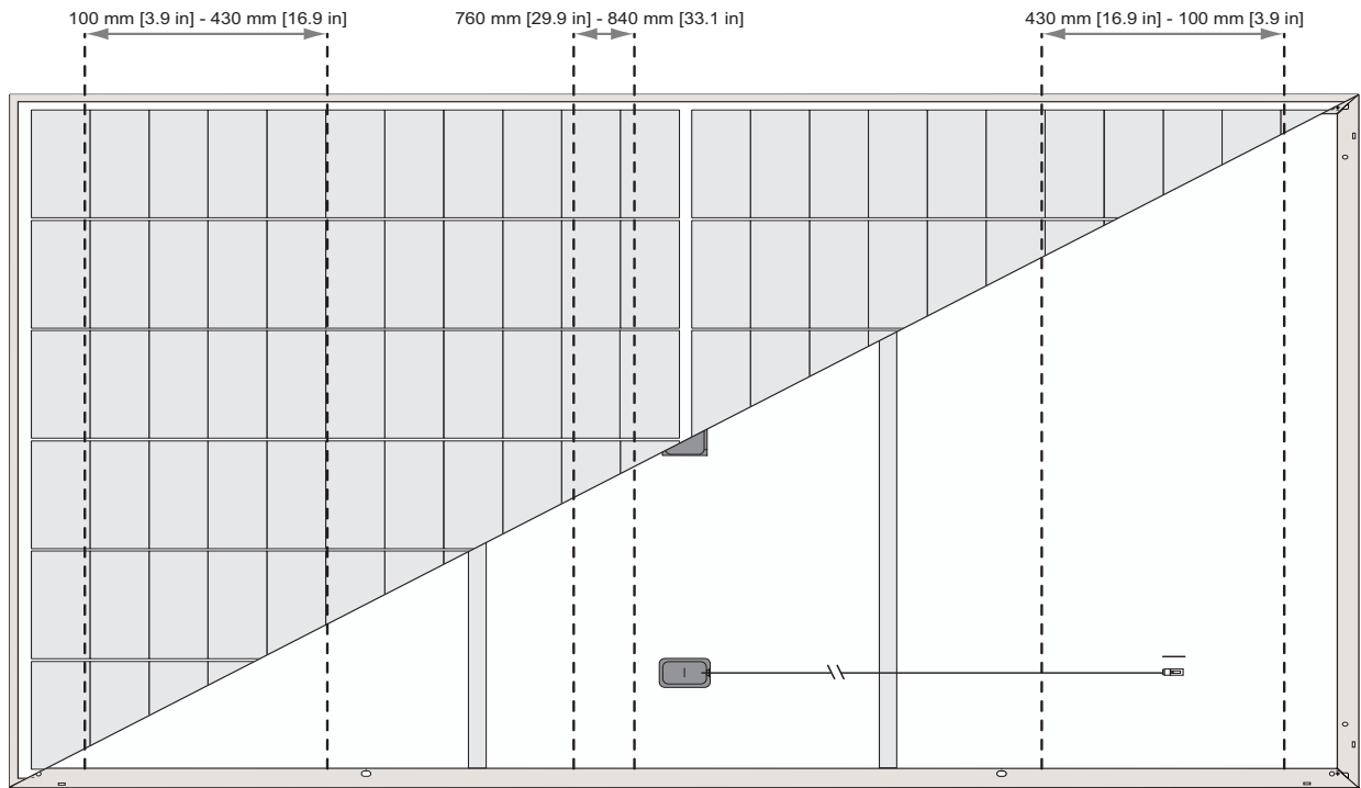
Fig. 2-4 Zonas de sujeción de la configuración de montaje de seis puntos: REC Alpha Pure Series
