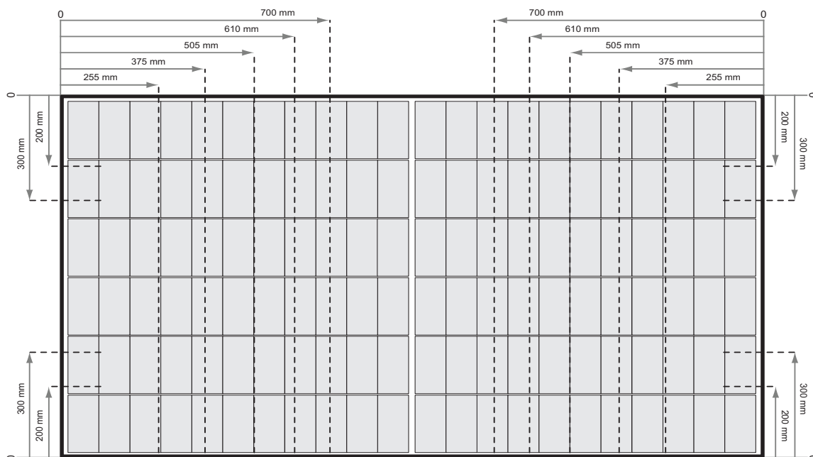
Fig. 2-1 Sujeción de paneles REC Alpha Pure Series con ralles paralelos al lado corto del panel
