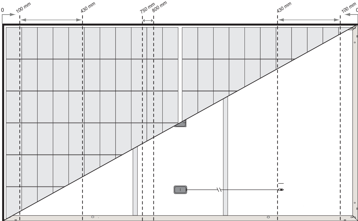
Fig. 3-4 Zonas de sujeción de la configuración de montaje de seis puntos: REC Alpha Pure 2 Series
