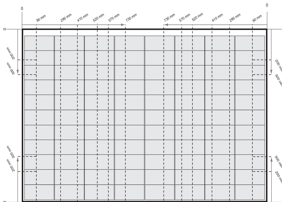
Fig. 5-1 Sujeción de paneles REC Alpha Pure-RX Series con raíles paralelos al lado corto del panel
