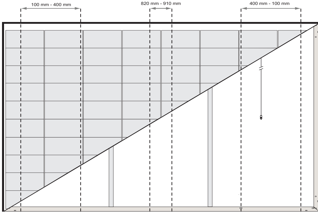
Fig. 4-4 Zonas de sujeción de configuración de montaje de seis puntos: REC Alpha Pure-R Series
