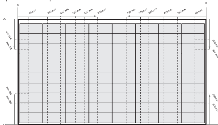
Fig. 4-3 Sujeción de los paneles REC Alpha Pure-R Series mediante raíles cortos
