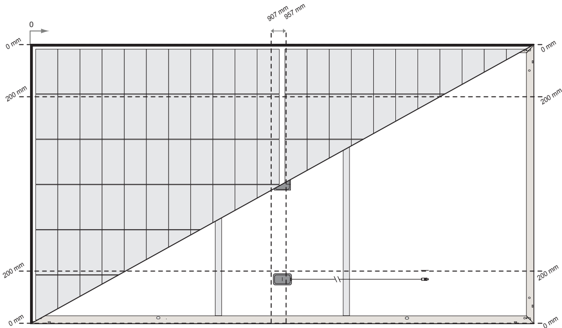
Fig. 3-5 Montaje mixto de seis puntos de los paneles REC Alpha Pure 2 Series utilizando carriles cortos
