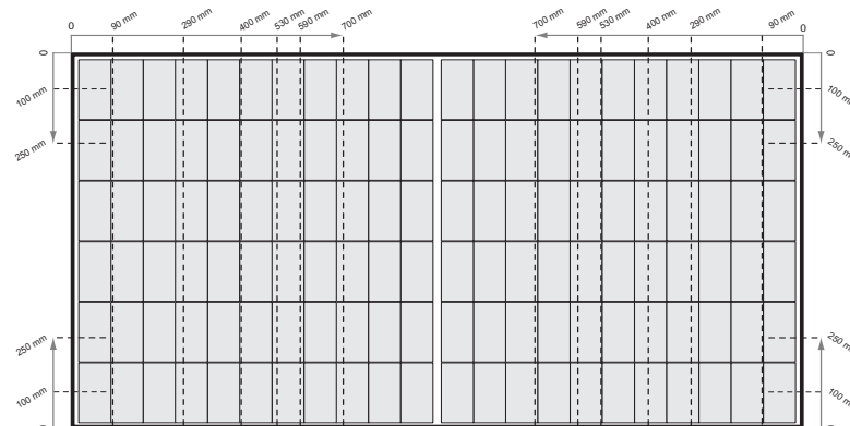
Fig. 3-3 Sujeción de los paneles REC Alpha Pure Series 2 mediante carriles cortos
