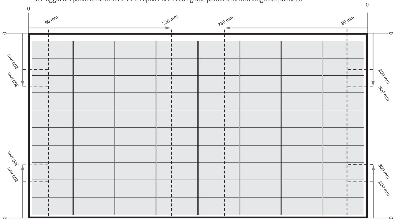
fig. 4-2 Serraggio dei pannelli della serie REC Alpha Pure-R con guide parallele al lato lungo del pannello
