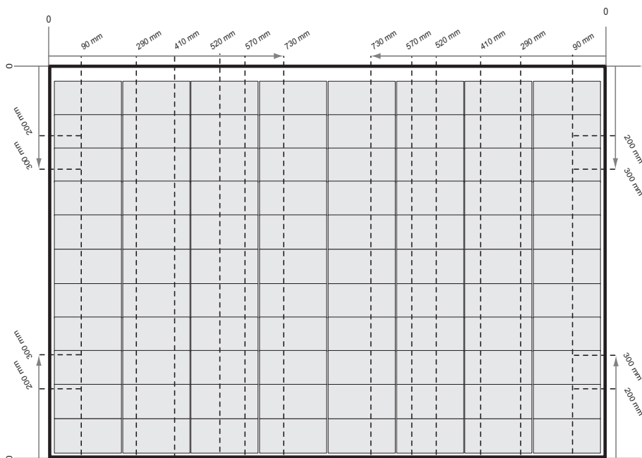
fig. 5-1 Serraggio dei pannelli della serie REC Alpha Pure-RX con guide parallele al lato corto del pannello
