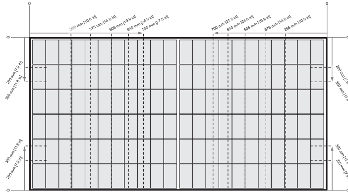
fig. 2-3 Serraggio dei pannelli REC Alpha Pure Series con binari corti
