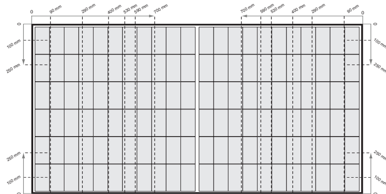
fig. 3-3 Serraggio dei pannelli della serie REC Alpha Pure 2 con guide corte
