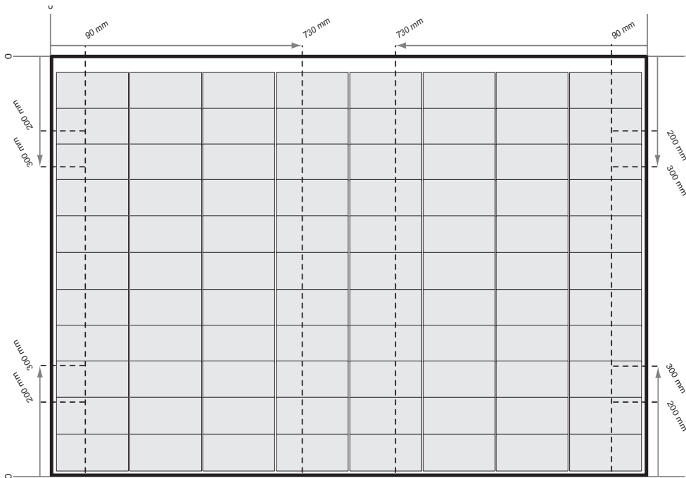
fig. 5-2 Serraggio dei pannelli della serie REC Alpha Pure-RX con guide parallele al lato lungo del pannello
