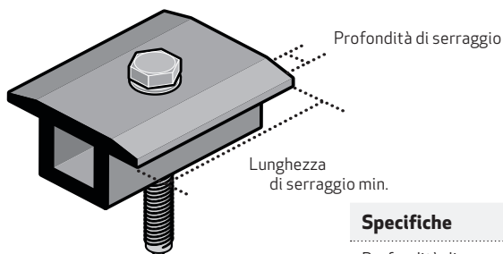
fig. 1 Specifiche del morsetto
