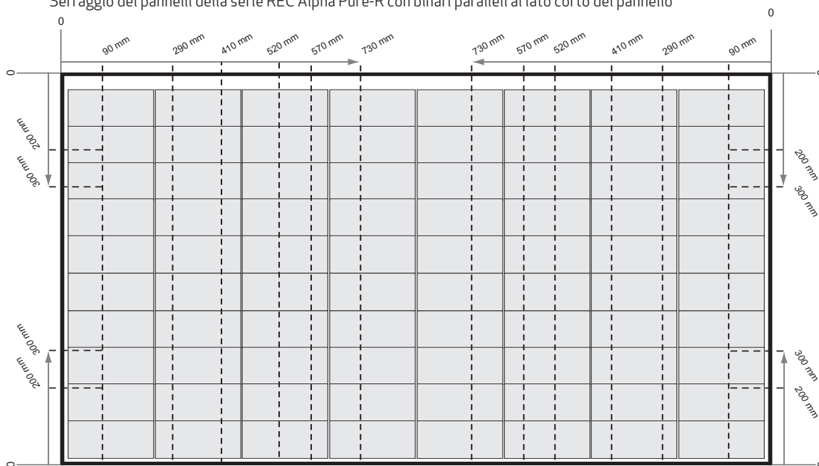
fig. 4-1 Serraggio dei pannelli della serie REC Alpha Pure-R con binari paralleli al lato corto del pannello
