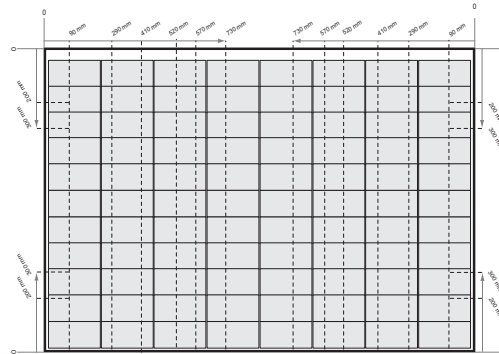
fig. 5-3 Serraggio dei pannelli della serie REC Alpha Pure-RX con binari corti
