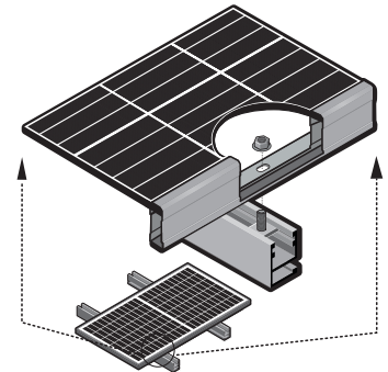
fig. 4 Esempio di installazione dei fori di montaggio
