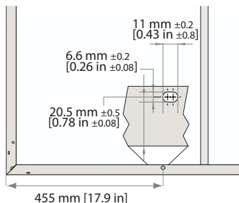
fig. 3 Fori di montaggio: Pannelli REC Alpha
