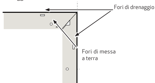
fig. 1-5 Fori di drenaggio e messa a terra
