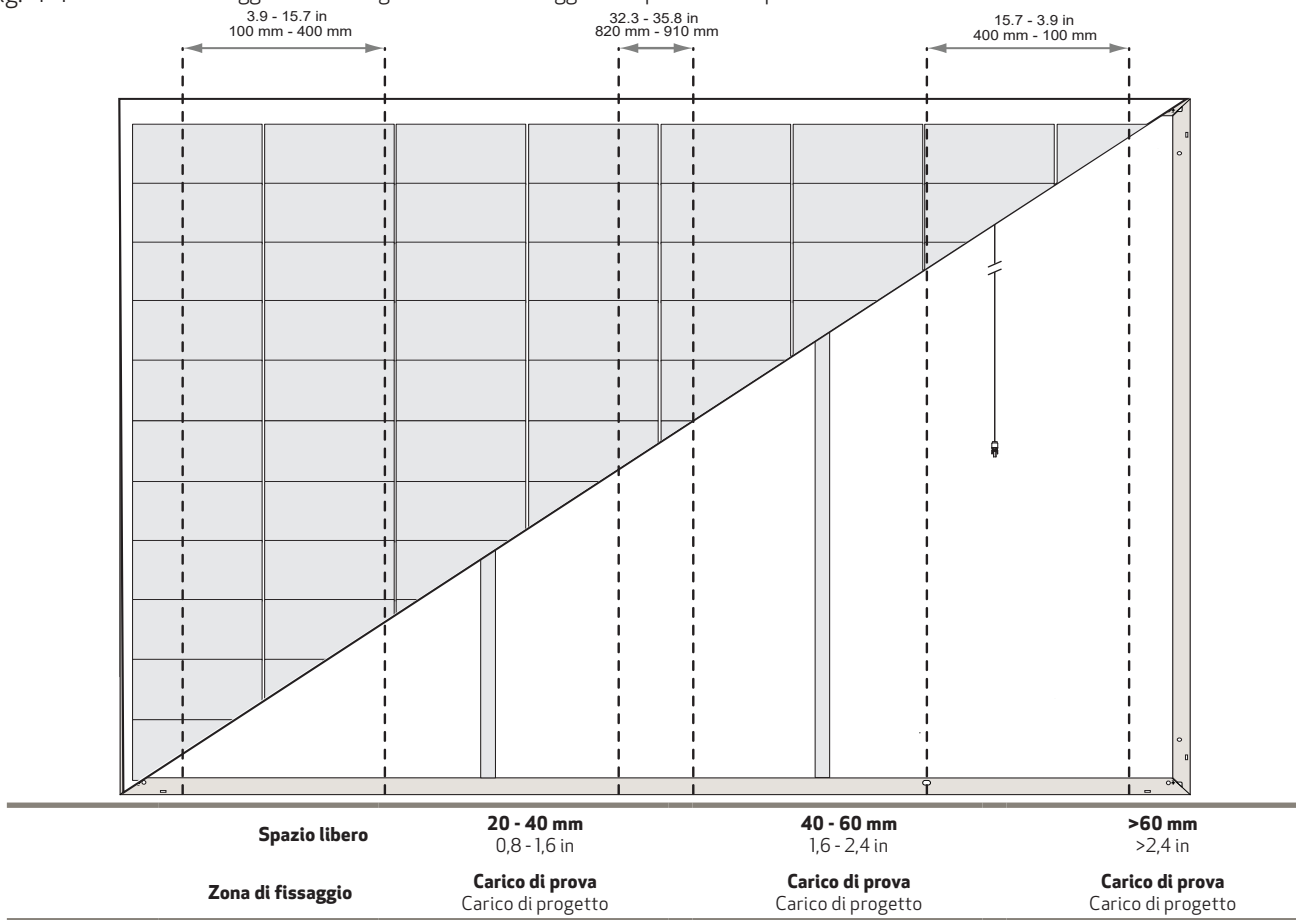
fig. 4-4 Zone di serraggio della configurazione di montaggio a sei punti: REC Alpha Pure-RX
