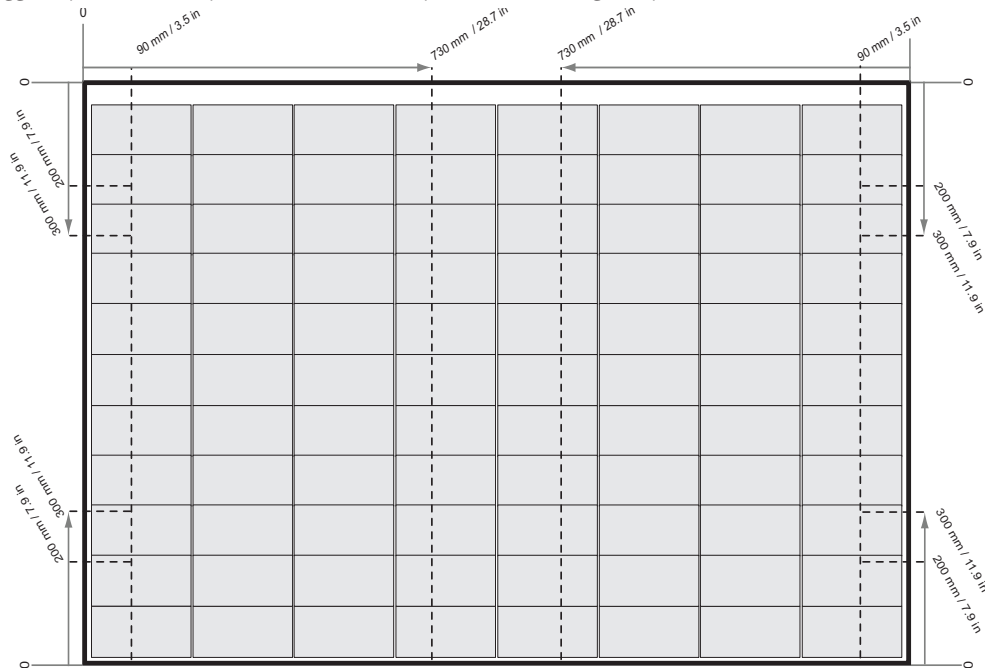
fig. 4-2 Serraggio di pannelli REC Alpha Pure-RX con binari paralleli al lato lungo del pannello
