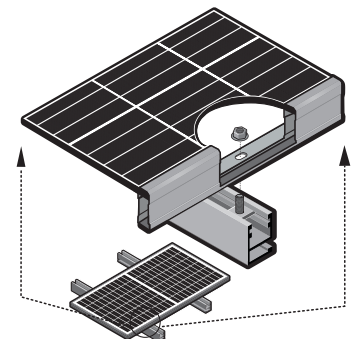
fig. 1-4 Esempio di installazione dei fori di montaggio
