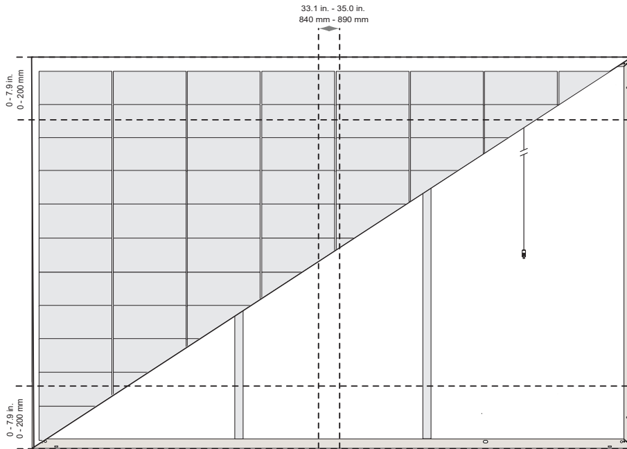
fig. 4-5 Montaggio misto a sei punti dei pannelli della serie REC Alpha Pure-RX con binari corti
