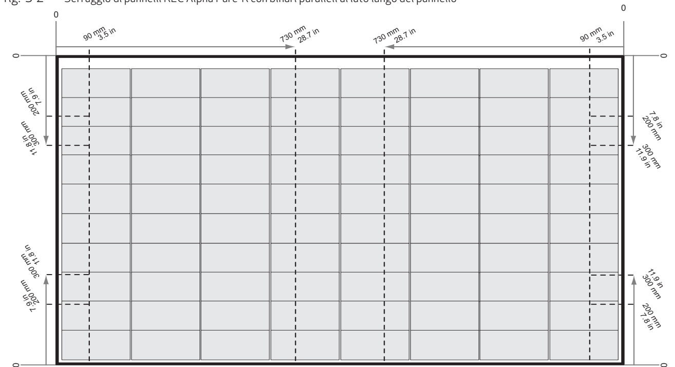
fig. 3-2 Serraggio di pannelli REC Alpha Pure-R con binari paralleli al lato lungo del pannello
