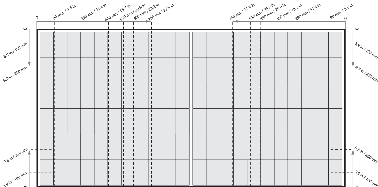
fig. 2-1 Serraggio di pannelli REC Alpha Pure 2 con binari paralleli al lato corto del pannello
