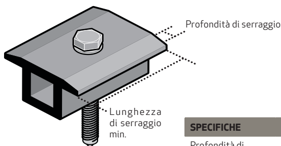
fig. 1-1 Specifiche del morsetto
