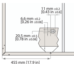
fig. 1-3 Fori di montaggio: Pannelli REC Alpha
