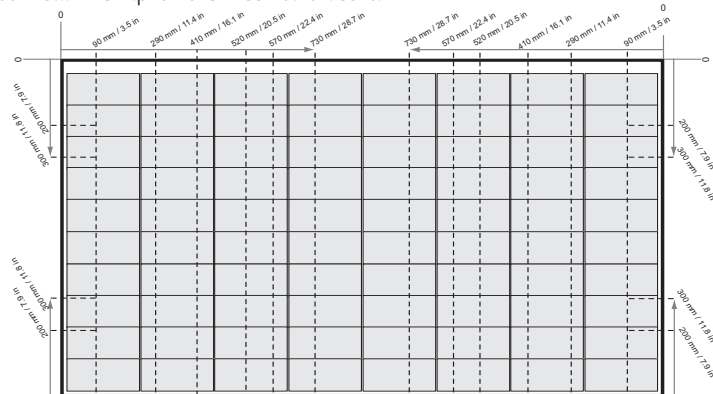
fig. 3-3 Serraggio di pannelli REC Alpha Pure-R con binari corti
