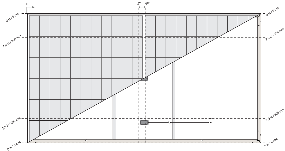
fig. 2-5 Montaggio misto a sei punti dei pannelli della serie REC Alpha Pure 2 con binari corti
