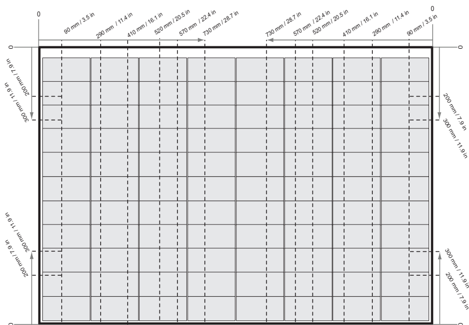
fig. 4-1 Serraggio di pannelli REC Alpha Pure-RX con binari paralleli al lato corto del pannello
