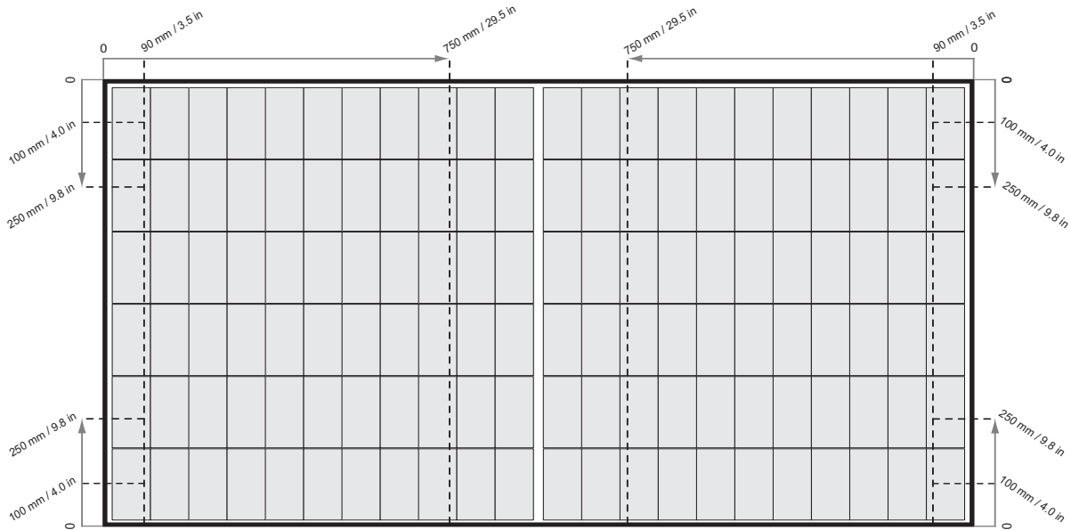
fig. 2-2 Serraggio di pannelli REC Alpha Pure 2 con binari paralleli al lato lungo del pannello
