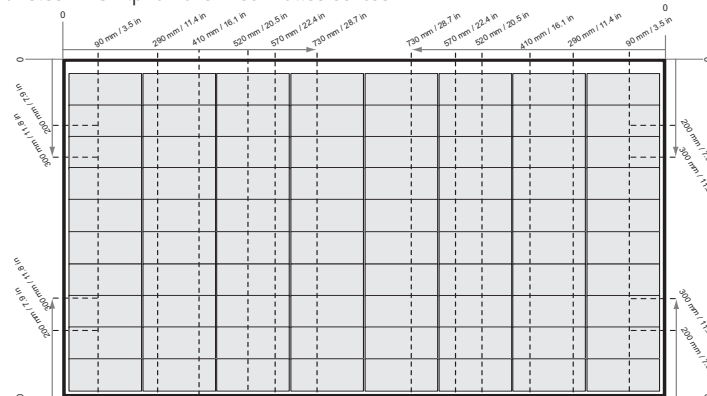
Fig. 3-3 Sujeción de paneles REC Alpha Pure-R con raíles cortos
