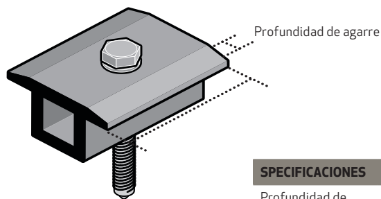
Fig. 1-1 Especificaciones de la abrazadera
