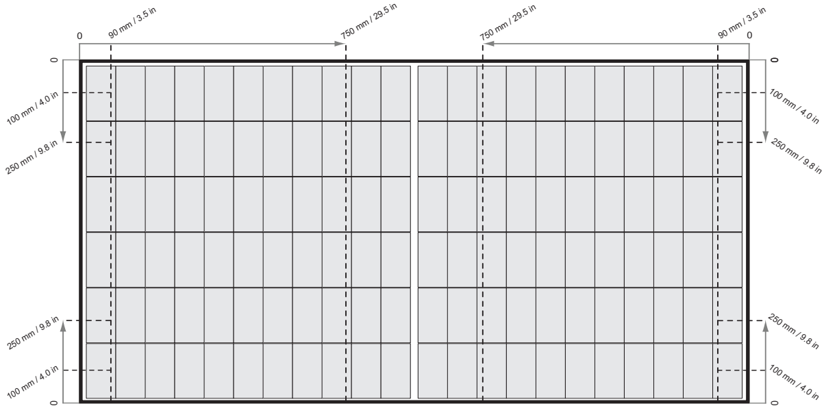
Fig. 2-2 Sujeción de paneles REC Alpha Pure 2 con ralles paralelos al lado largo del panel
