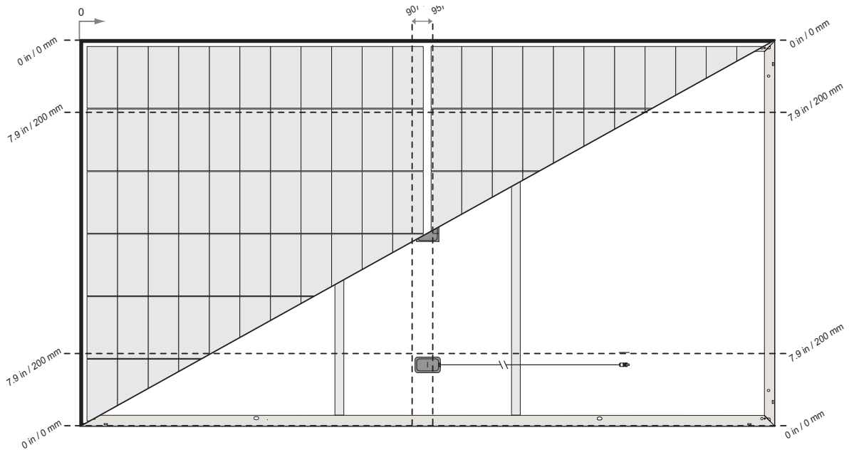
Fig. 2-5 Montaje mixto de seis puntos de los paneles de la serie REC Alpha Pure 2 utilizando raíles cortos
