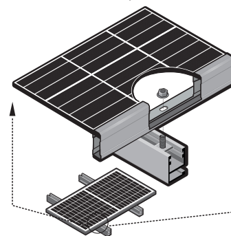
Fig. 1-4 Ejemplo de instalación de orificios de montaje
