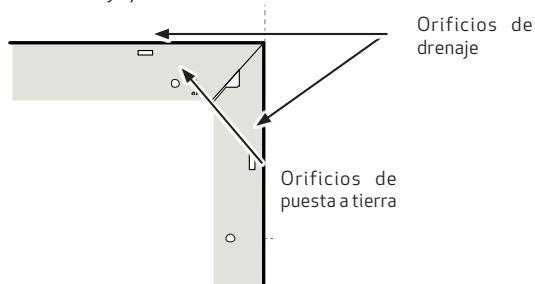
Fig. 1-5 Orificios de drenaje y conexión a tierra
