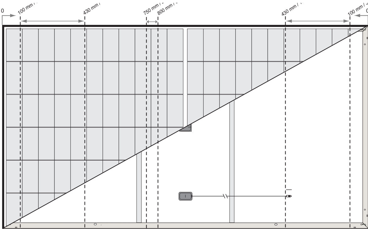
Fig. 2-4 Zonas de sujeción de la configuración de montaje de seis puntos: REC Alpha Pure 2
