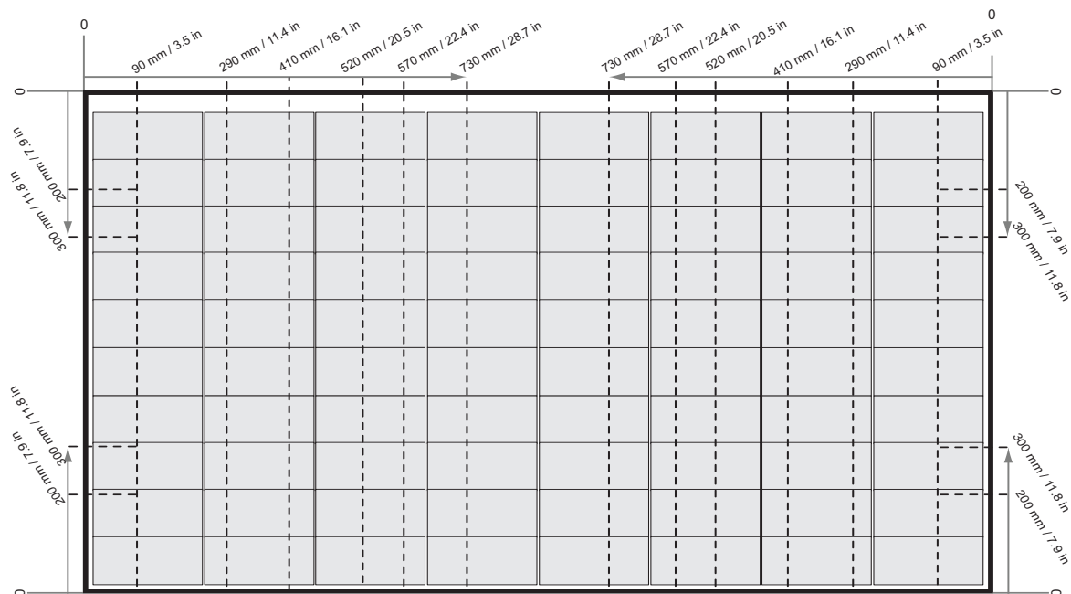
Fig. 3-1 Sujeción de paneles REC Alpha Pure-R con riles paralelos al lado corto del panel
