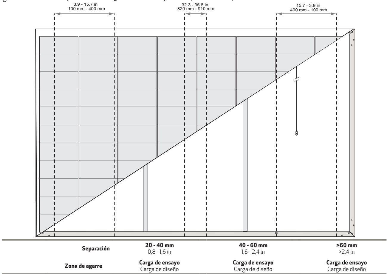
Fig. 4-4 Zonas de sujeción de la configuración de montaje de seis puntos: REC Alpha Pure-RX
