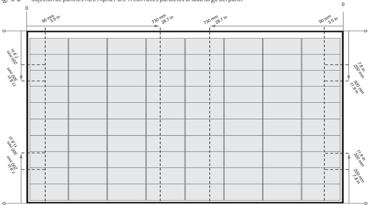
Fig. 3-2 Sujeción de paneles REC Alpha Pure-R con raíles paralelos al lado largo del panel
