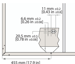
Fig. 1-3 Orificios de montaje: Paneles REC Alpha
