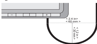
Fig. 1-6 Distancia mínima del cable
