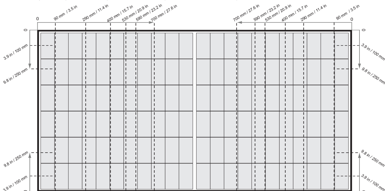
Fig. 2-1 Sujeción de paneles REC Alpha Pure 2 con ralles paralelos al lado corto del panel
