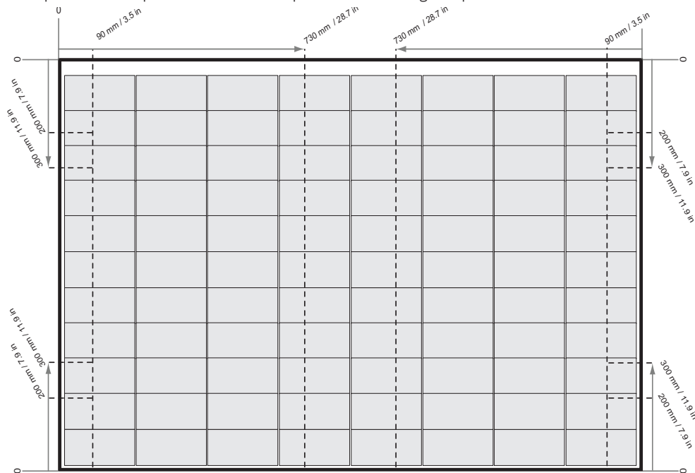
Fig. 4-2 Sujeción de paneles REC Alpha Pure-RX con raíles paralelos al lado largo del panel
