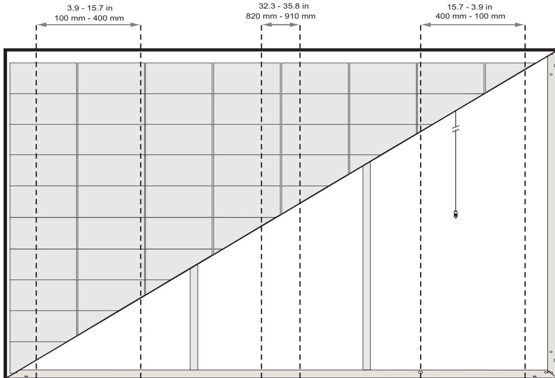
Fig. 3-4 Zonas de sujeción de la configuración de montaje de seis puntos: REC Alpha Pure-R
