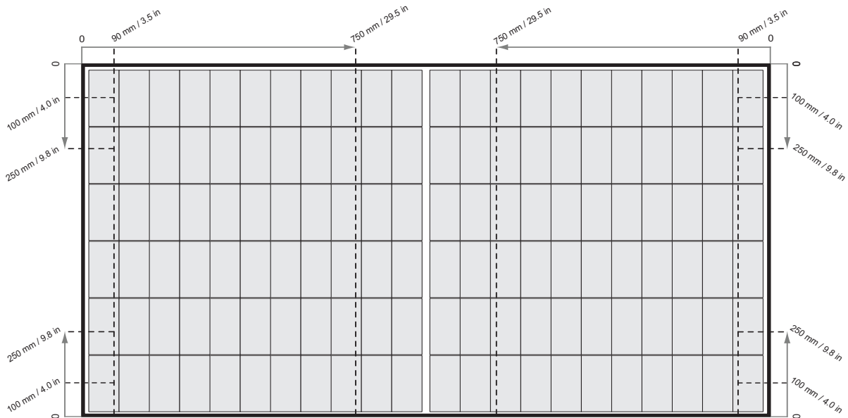
図 2-2 パネルの長辺と平行なレールを使用した REC Alpha Pure 2 パネルのクランプ
