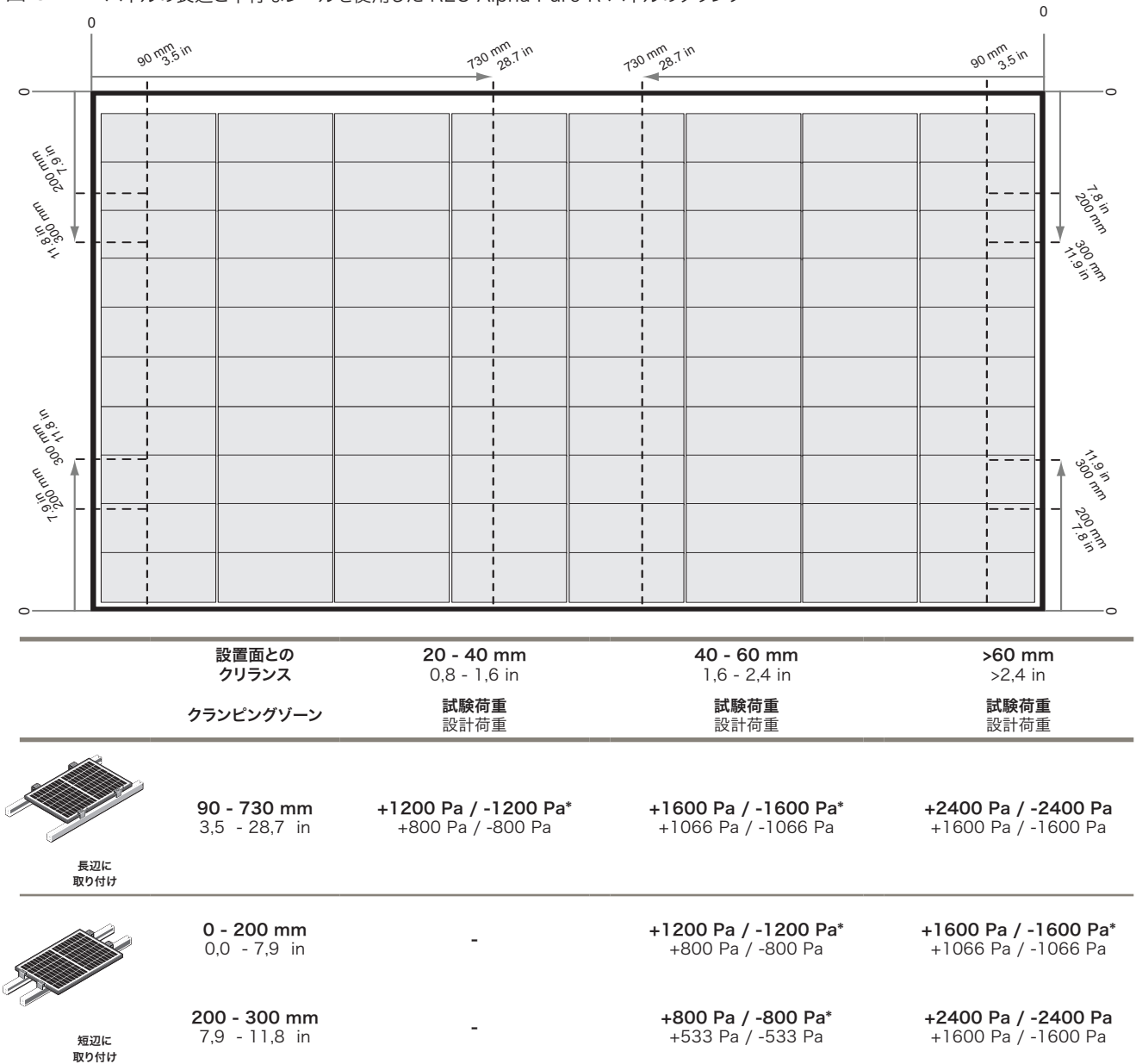
図 3-2 パネルの長辺と平行なレールを使用した REC Alpha Pure-R パネルのクランプ
