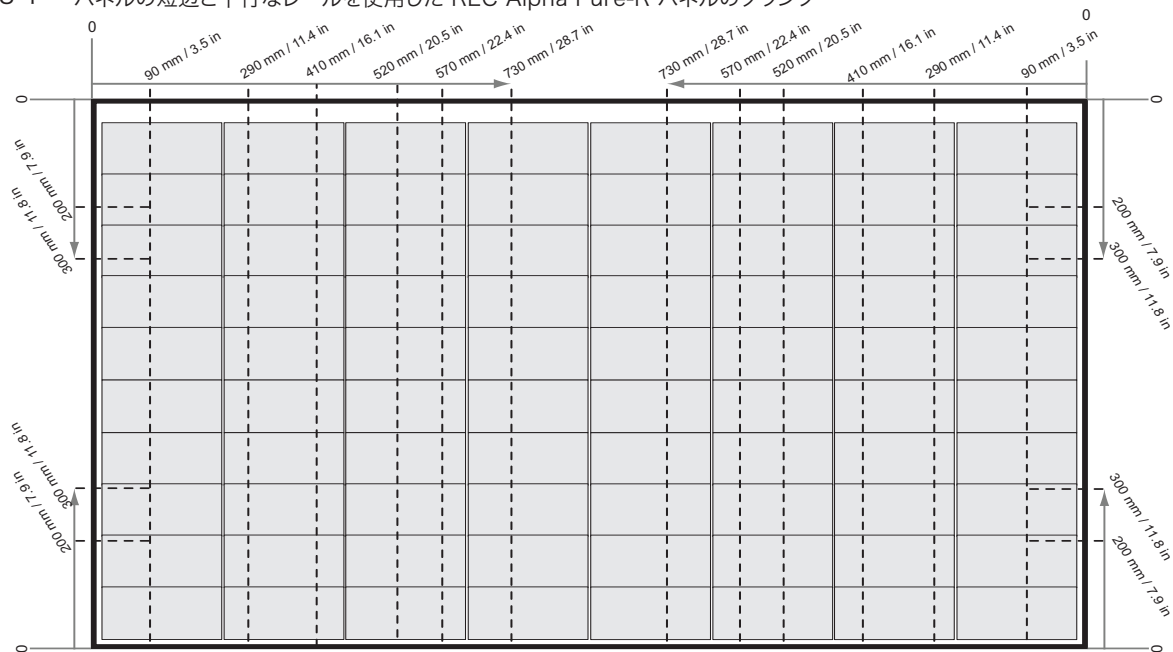
図 3-1 パネルの短辺と平行なレールを使用した REC Alpha Pure-R パネルのクランプ
