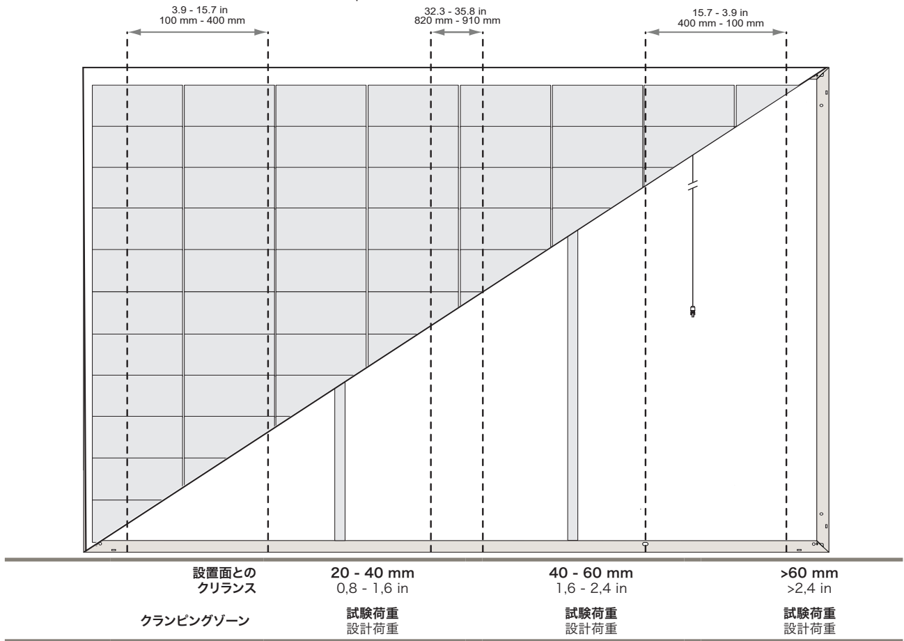
図 4-4 6点取り付け構成クランピングゾーン: REC Alpha Pure-RX
