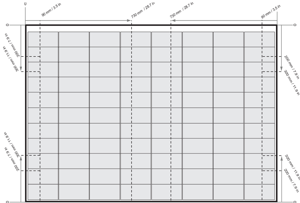
図 4-2 パネルの長辺と平行なレールを使用した REC Alpha Pure-RX パネルのクランプ
