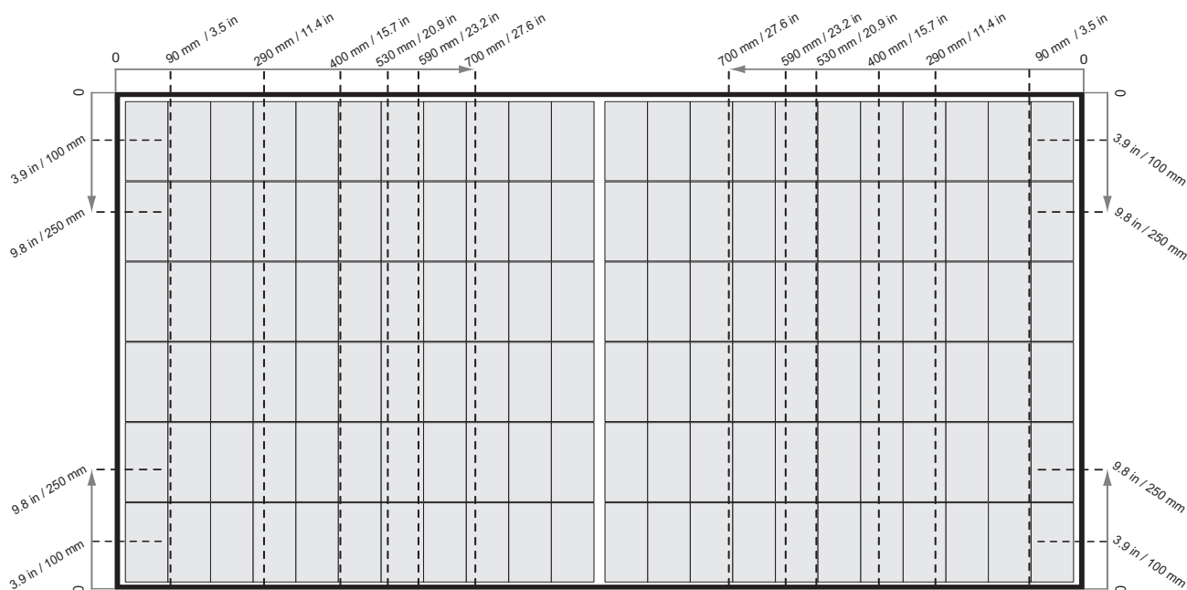
図 2-1 パネルの短辺と平行なレールを使用した REC Alpha Pure 2 パネルのクランプ
