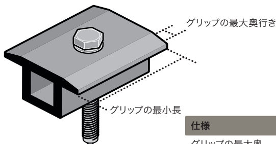
図1-1 クランプの仕様
