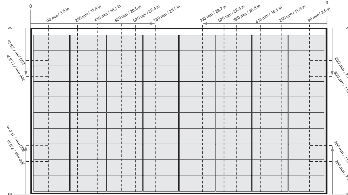
図 3-3 ショートレールを使用した REC Alpha Pure-R パネルのクランプ
