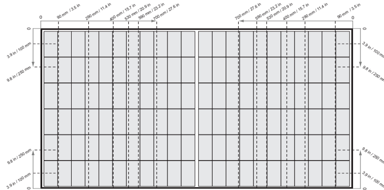
図 2-3 ショートレールを使用した REC Alpha Pure 2 パネルのクランプ
