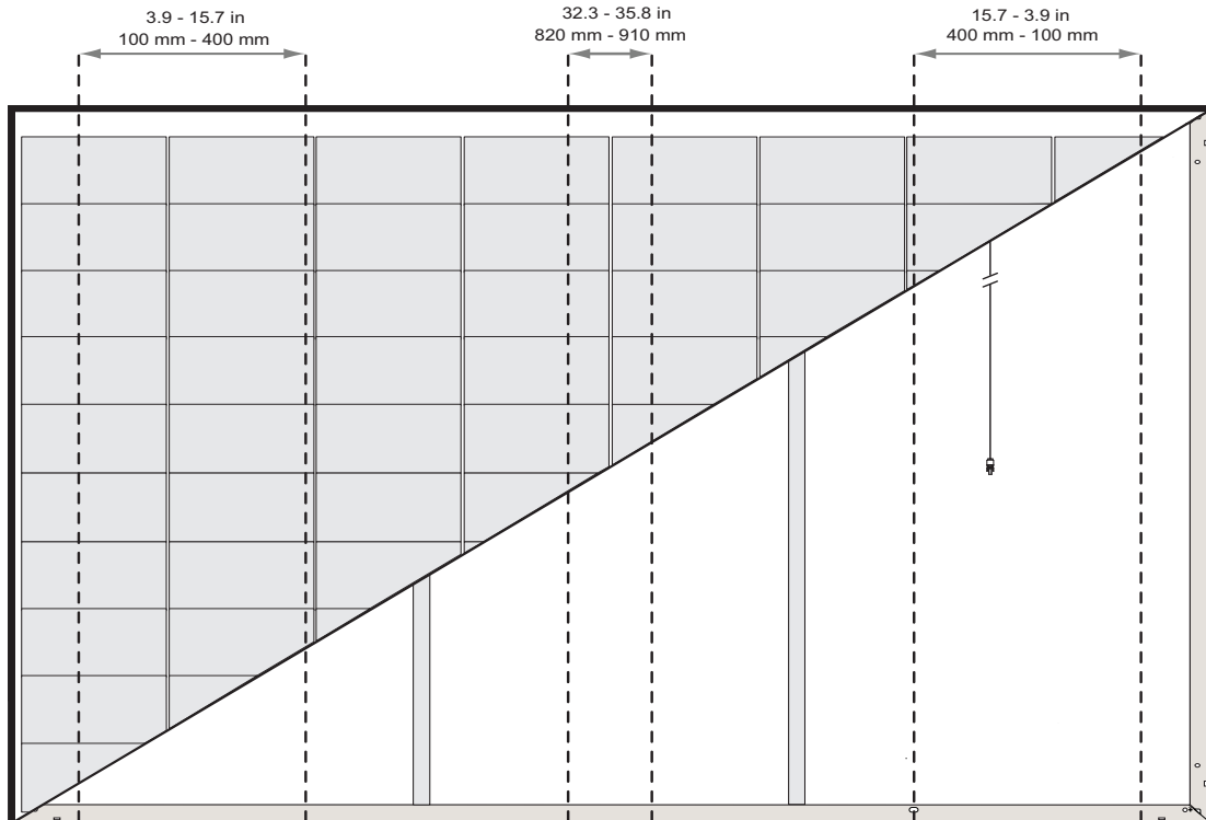
図 3-4 6点取り付け構成クランプゾーン: REC Alpha Pure-R
