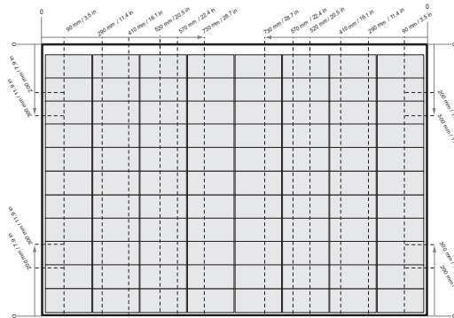
図 4-3 ショートレールを使用した REC Alpha Pure-RX パネルのクランプ
