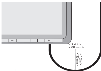
図1-6 ケーブルの最小曲げ半径
