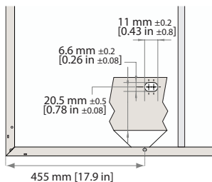
図1-3 取り付け穴:REC Alpha
