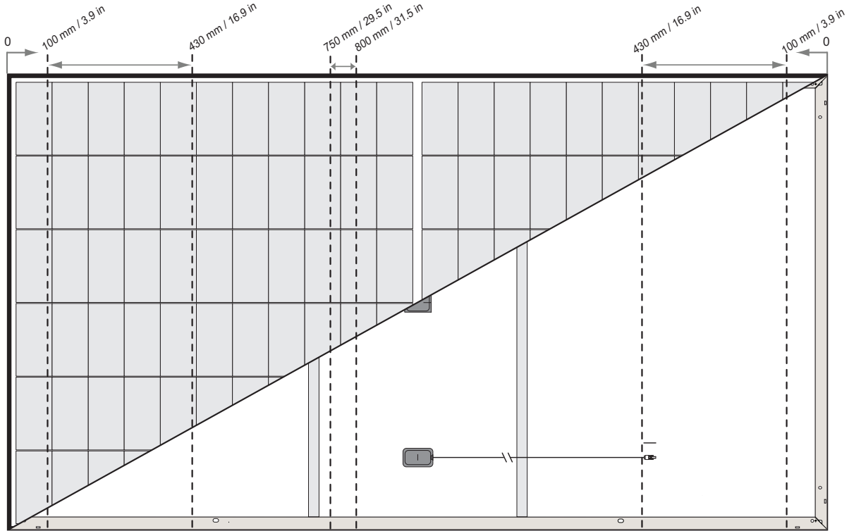
図 2-4 6点取り付け構成クランピングゾーン: REC Alpha Pure 2
