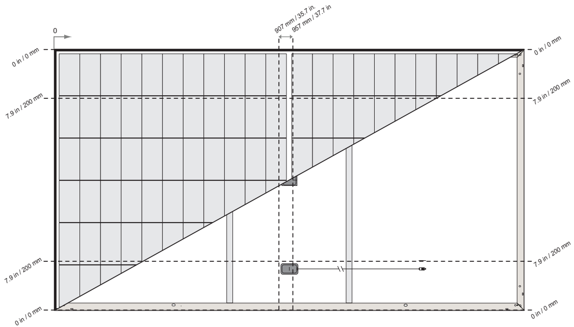
図 2-5 ショートレールを使用した REC Alpha Pure 2 シリーズ パネルの混合 6 点取り付け
